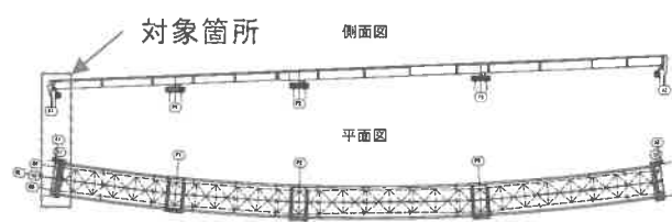
図-2 構造一般図
