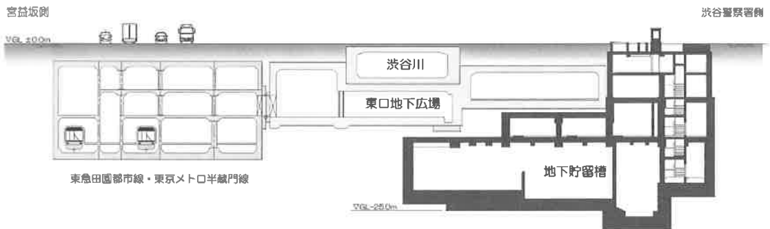
図-2 地下3施設断面図
