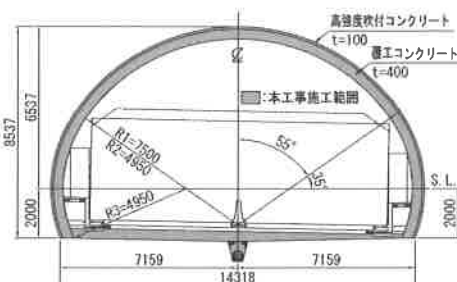
図ー1 標準断面図（標準部C II—VEパターン）
