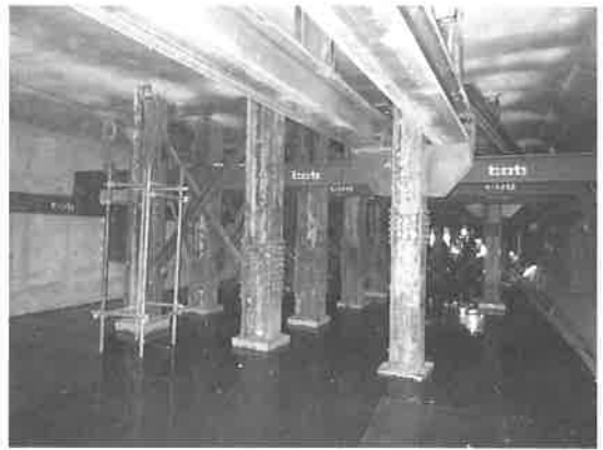
図－7 束立て工法状況
