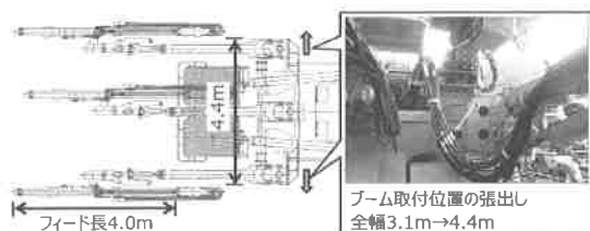
図-2 ドリルジャンボの改造 （削孔範囲の拡大およびフィーダ長の延長）
