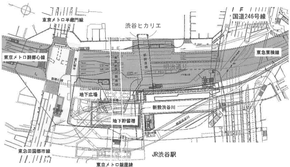
図-1 渋谷駅東口平面図
