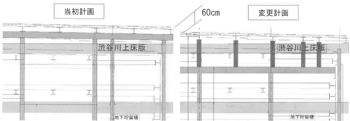
図－6 束立法による覆工高さの変更（側面図）
