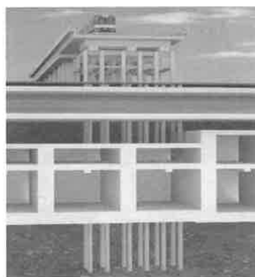
図4-2 銀座線仮受け
